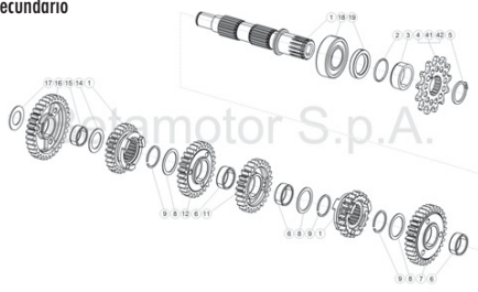
TAV.04B Albero secondario - Counter shaft - Arbre secondaire - Nebengetriebewelle - Eje secundario
