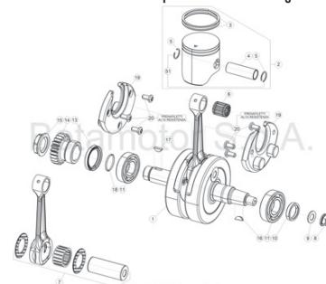
TAV.02 Albero motore - Crankshaft - Vilebrequin - Kurbelwelle - Cigüeñal
