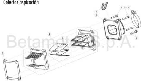
TAV.01C Collettore aspirazione - Intake manifold - Collecteur aspiration - Ansaugstutzen - Colector aspiración
