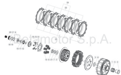
TAV.03 Frizione - Clutch - Embrayage - Kupplung - Embrague
