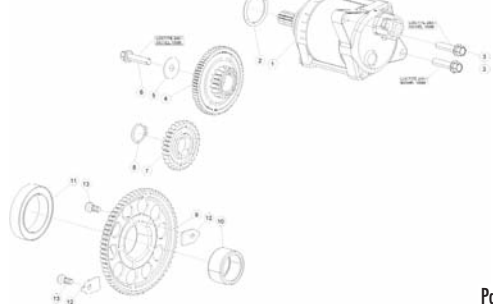
TAV.07 Avviamento elettrico - Electric starter - Dé marrage électrique - Elektrischer start - Arranque eléctrico
