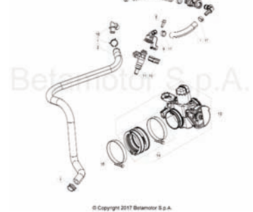
TAV.13 Gruppo iniezione - Injection unit - Groupe injection - Einspritzung - Grupo iniección
